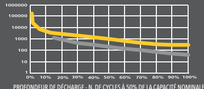
CYCLES DE VIE VS. PROFONDEUR DE DÉCHARGE POUR LES BATTERIES OPTIMA
