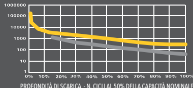
CICLI DI VITA CONTRO PROFONDITÀ DI SCARICA PER BATTERIE OPTIMA
